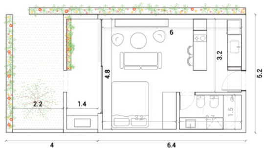
PLANTA ESQUEMÁTICA
